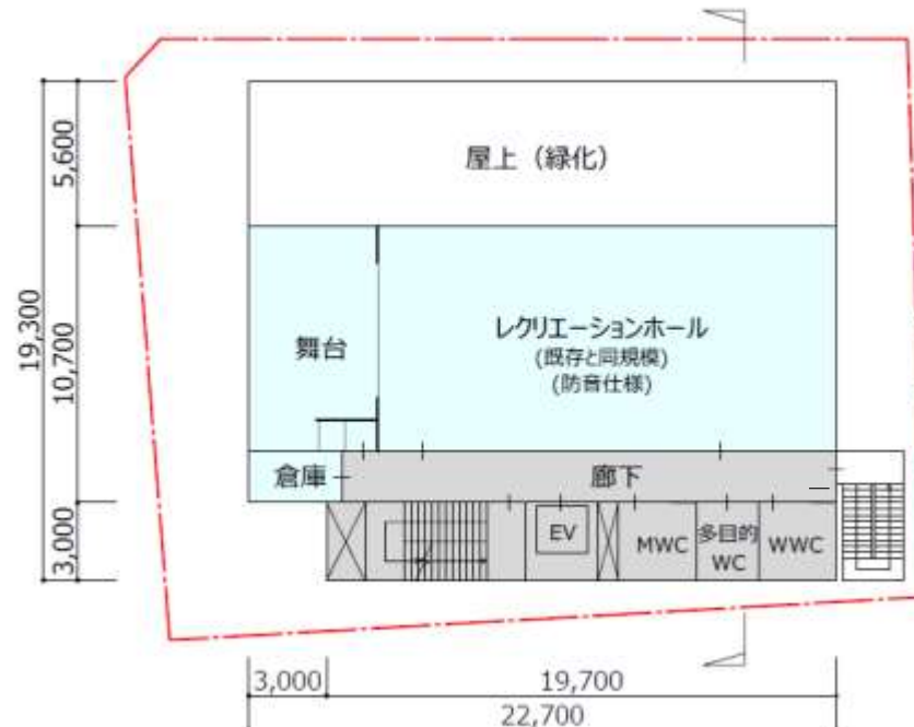
■ 3 階平面図
