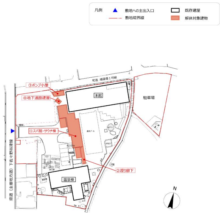
■ 解体対象建物範囲 (S : 1/800)
