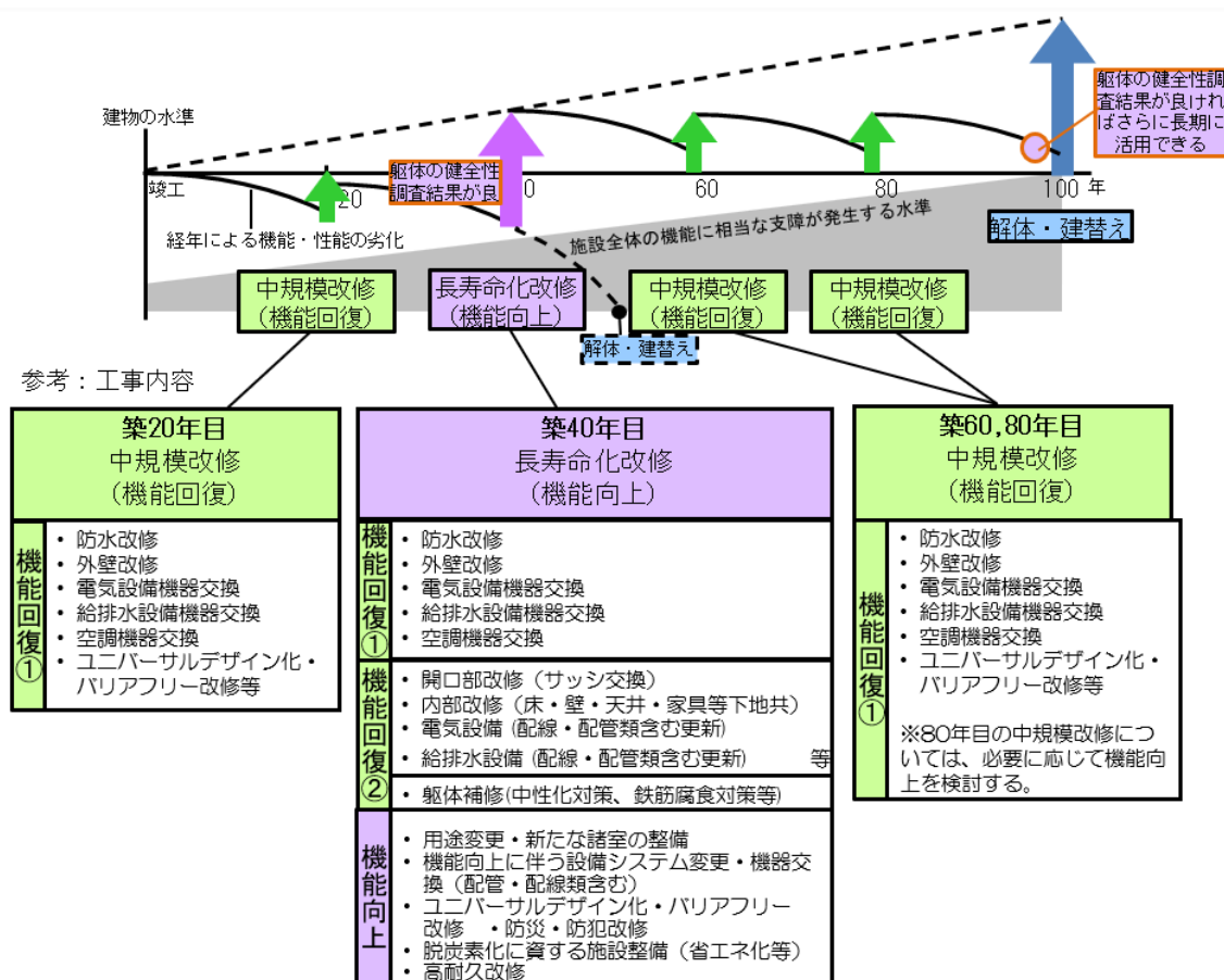
【表 5-3 計画的な保全による長寿命化の考え方※100 年の場合】
