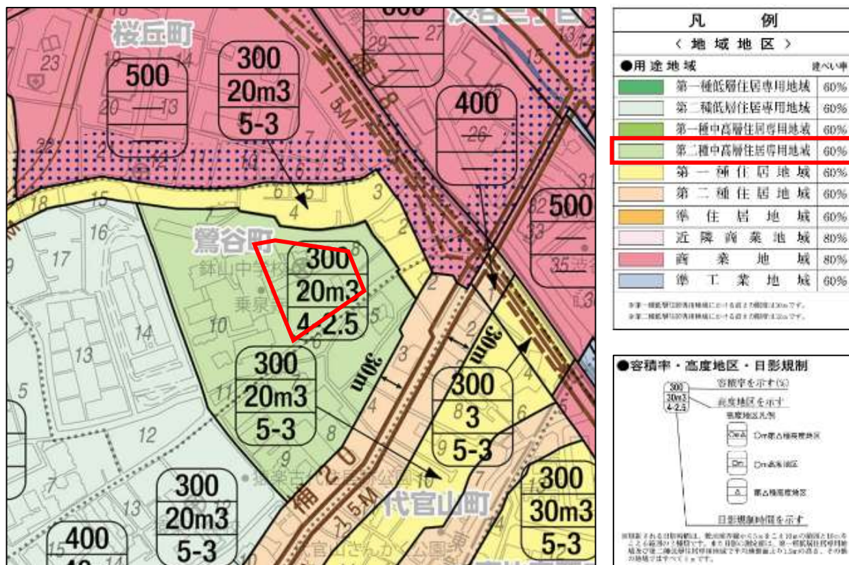
図Ⅱ-1-4 都市計画図(用途地域・高度地区)
