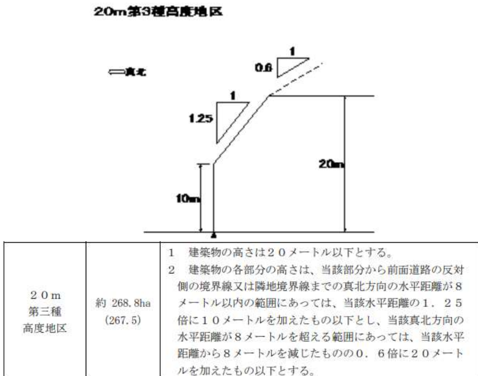
図Ⅱ-1-6 高度地区の解説
