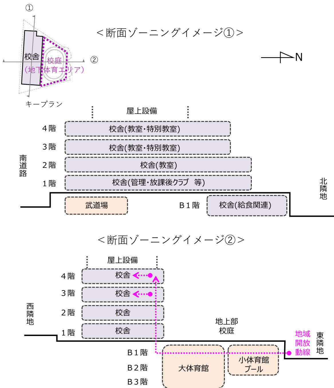
図V-2-5 断面計画パターン案
