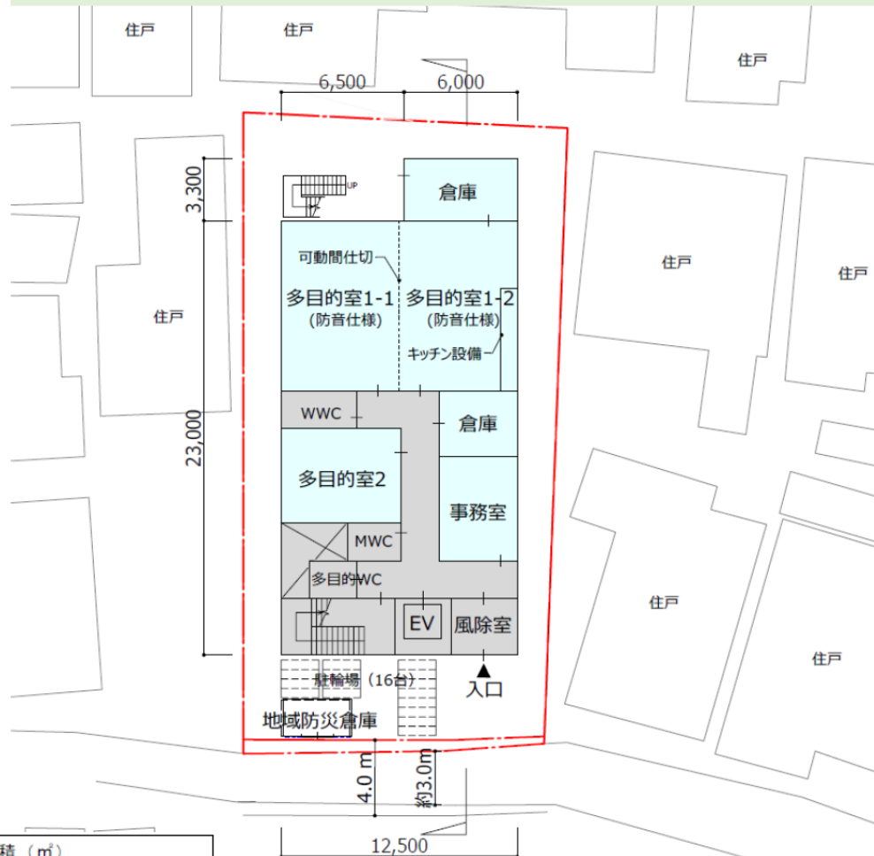
■ 配置兼1階平面図
