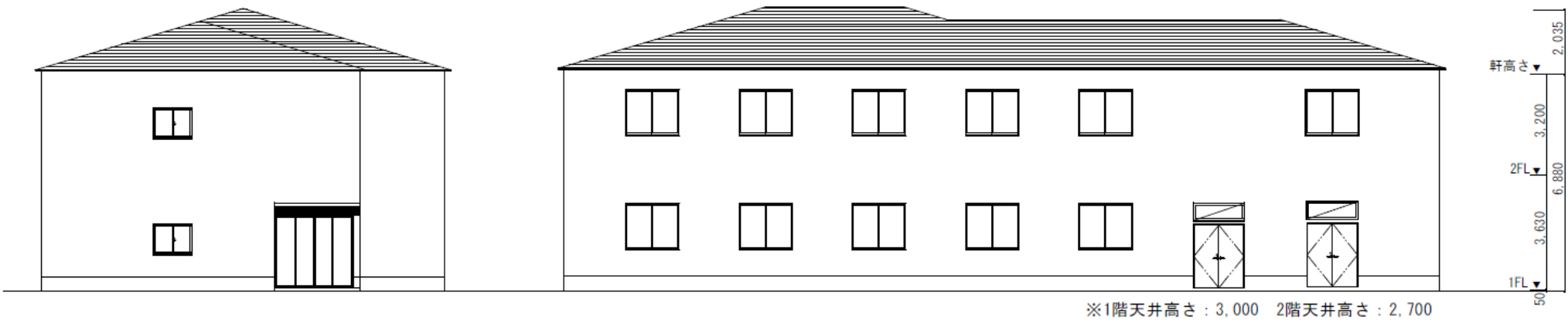
南側立面図
