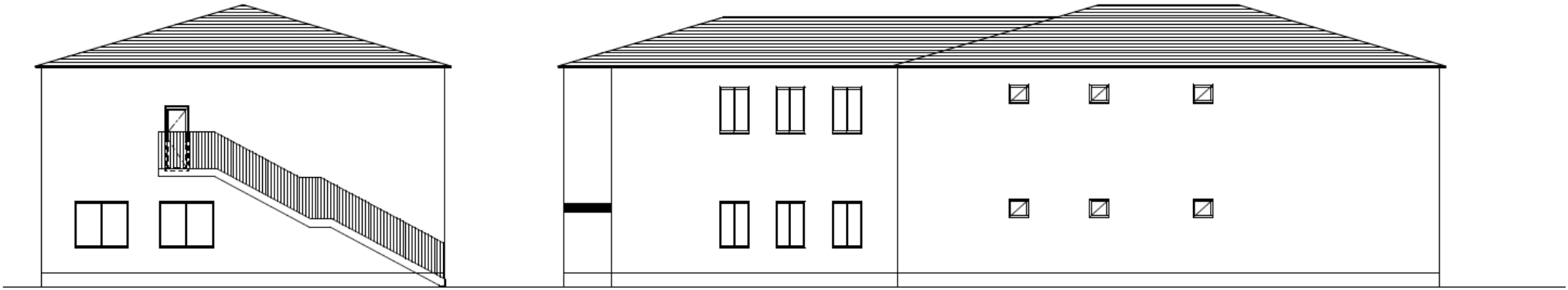
北側立面図
